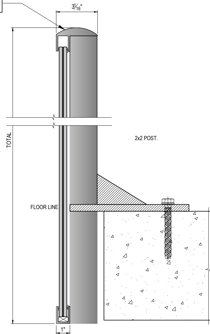
2 SECTION P16 SCALE: 6"=1'-0"
